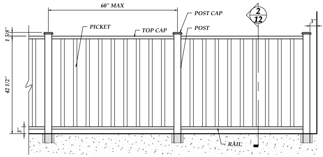
1 12 GUARDRAIL ELEVATION SCALE: 3/4"=1'-0"
