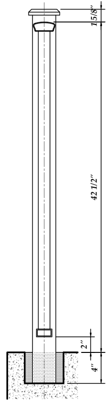
2 12 GUARDRAIL SECTION SCALE: 1-1/2"=1'-0"
