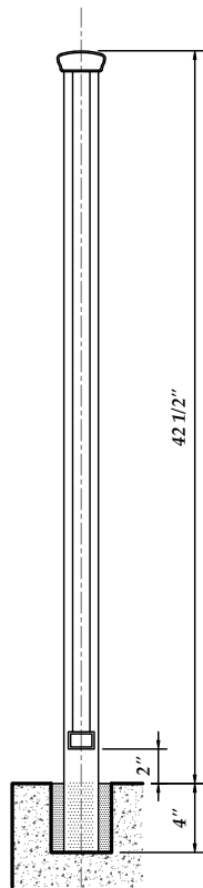
2 11 GUARDRAIL SECTION SCALE: 1-1/2"=1'-0"
