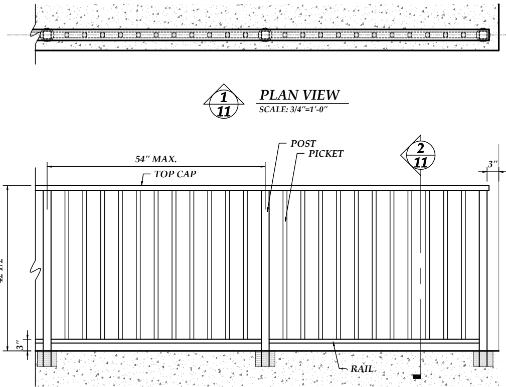
1 11 GUARDRAIL ELEVATION SCALE: 3/4"=1'-0"
