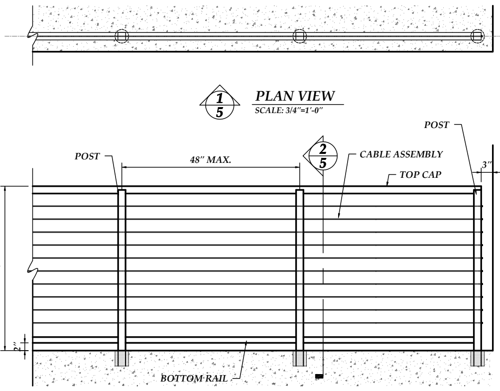
1 5 GUARDRAIL ELEVATION SCALE: 3/4"=1'-0"
